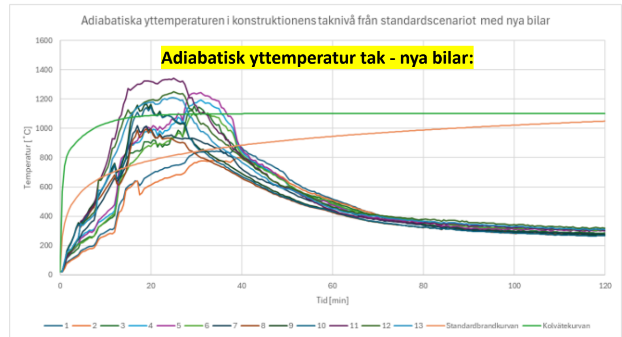
Figur 12. Temperatur-tidkurvor för brandpåverkan från nya fordon.
