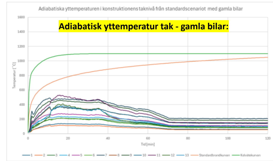
Figur 11. Temperatur-tidkurvor för brandpåverkan från gamla fordon.
