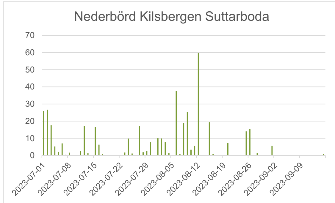
Figur 4. Nederbördsdata från SMHI:s mätstation Kilsbergen Suttarboda i Örebro kommun, från 1 juli till 15 september 2023.
