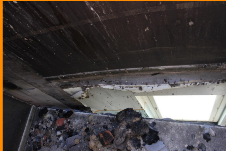
Golvbjälklag i trapphus
